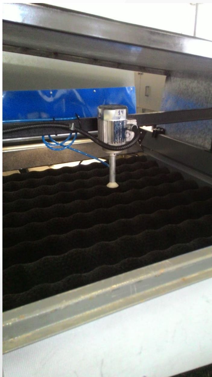
Aplicador de cera com sistema orbital
